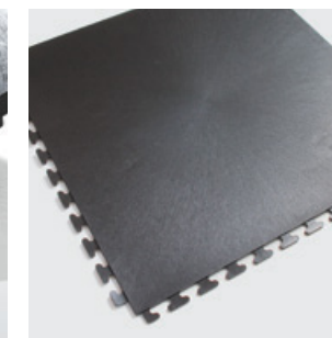
WALastic Clip dlaždice 500 x 500 mm Hrúbka: 6 mm Povrch: zrnitý/R11
